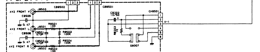
AV FRONT P. C. Board
