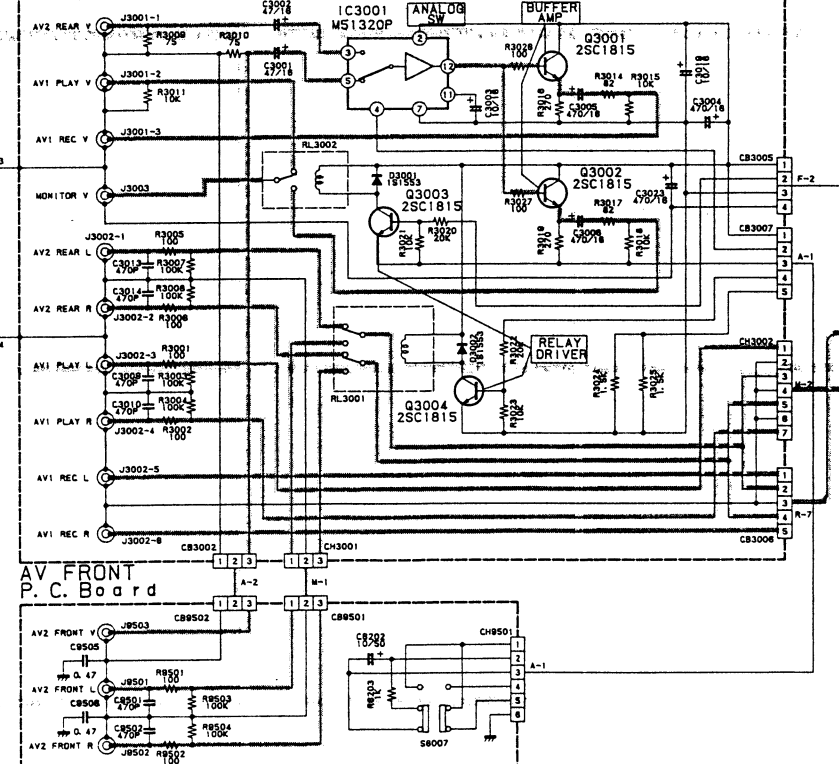
AV MONITOR P. C. Board
